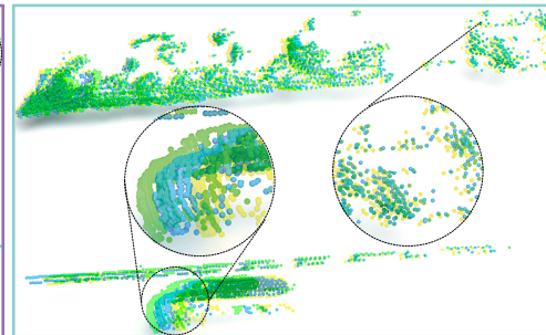
GMSF
